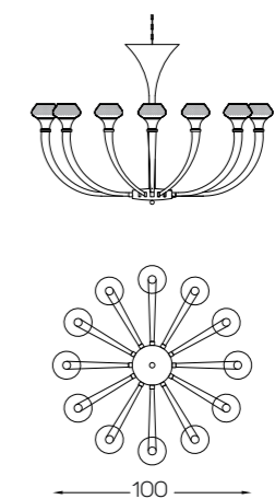
Art.1946/CH12/NL H 80 cm ø 100 cm 12 x E14 x 40W
