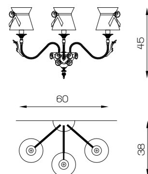
Art.1850/A3 H 45 cm L 60 cm Sp 38 cm 3 x E14 x 40W
