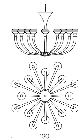
Art.1946/CH16/NL H 80 cm ø 130 cm 16 x E14 x 40W
