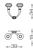
Art.1946/A2/NL H 34 cm L 39 cm Sp 19 cm 2 x E14 x 40W
