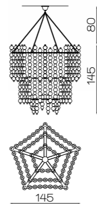
Art.1980/LU/TR H 145 cm ø 145 cm + 80 cm chain 30 x E14 x 40W
